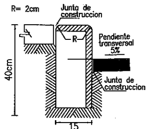
GUARNICION TIPO "I"
