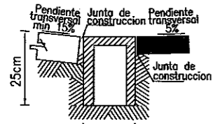
GUARNICION TIPO PATIN PARA COCHERA
